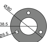
7038 90x38.5 □ 4
