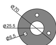
7025 70x25.5 □ 4
