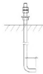
Анкер будівельний
